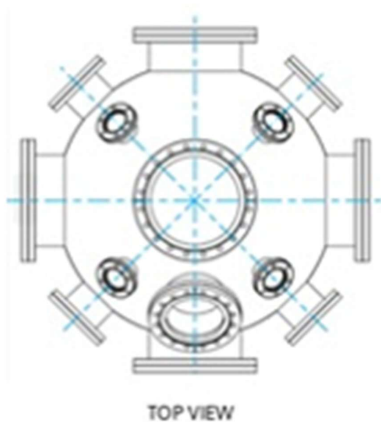
Obr. 2 – Pohled shora
