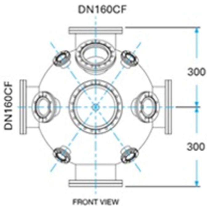
Obr. 3 – Pohled čelní
