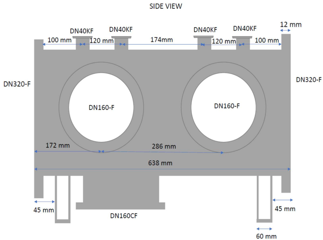
Obr. 1 – Pohled boční
