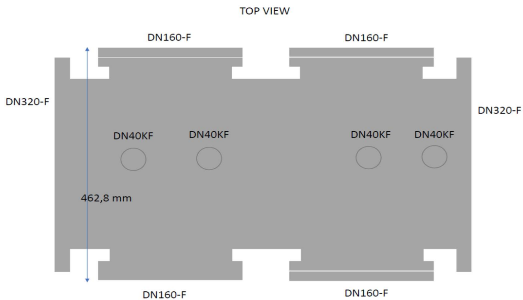
Obr. 2 – Pohled shora
